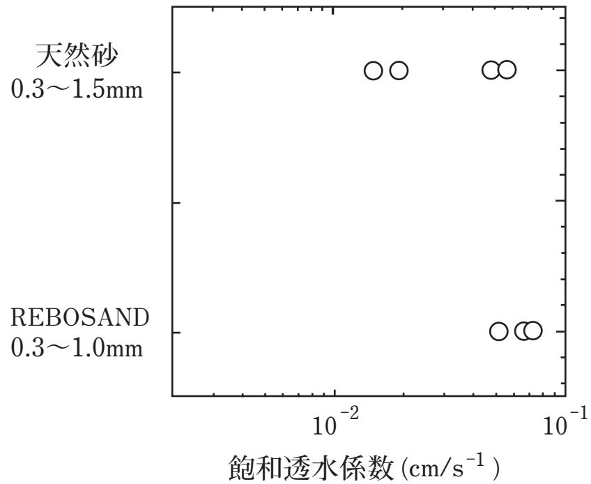
図1 飽和透水試験の測定結果(試料数：天然砂のみ4,その他は3)
